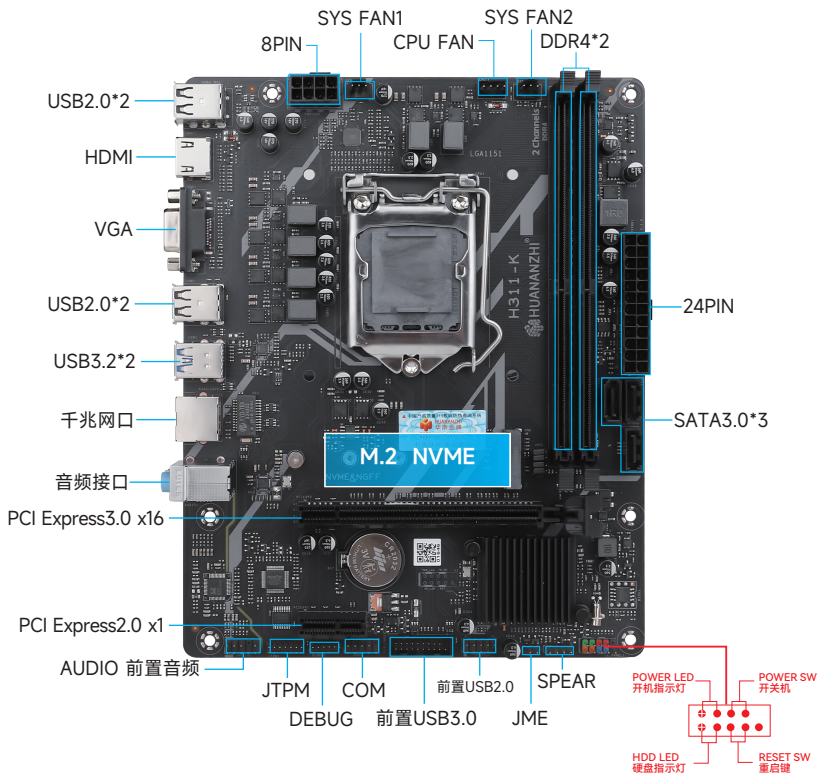
图1-1 H311-K主板图解
