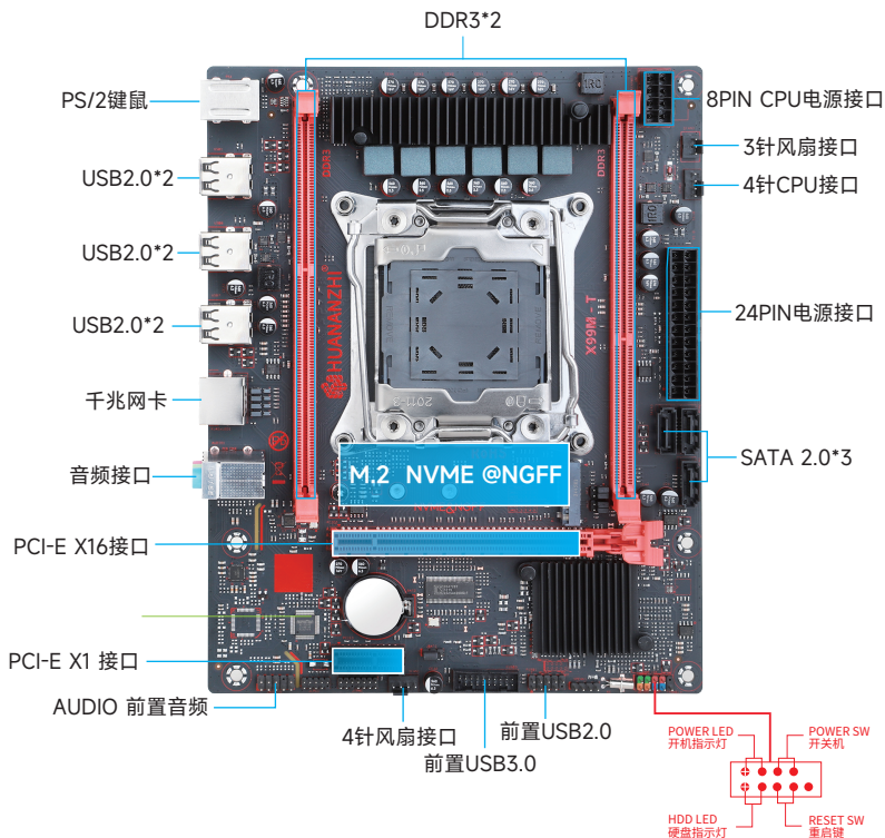
图1-1 X99M-T主板图解
