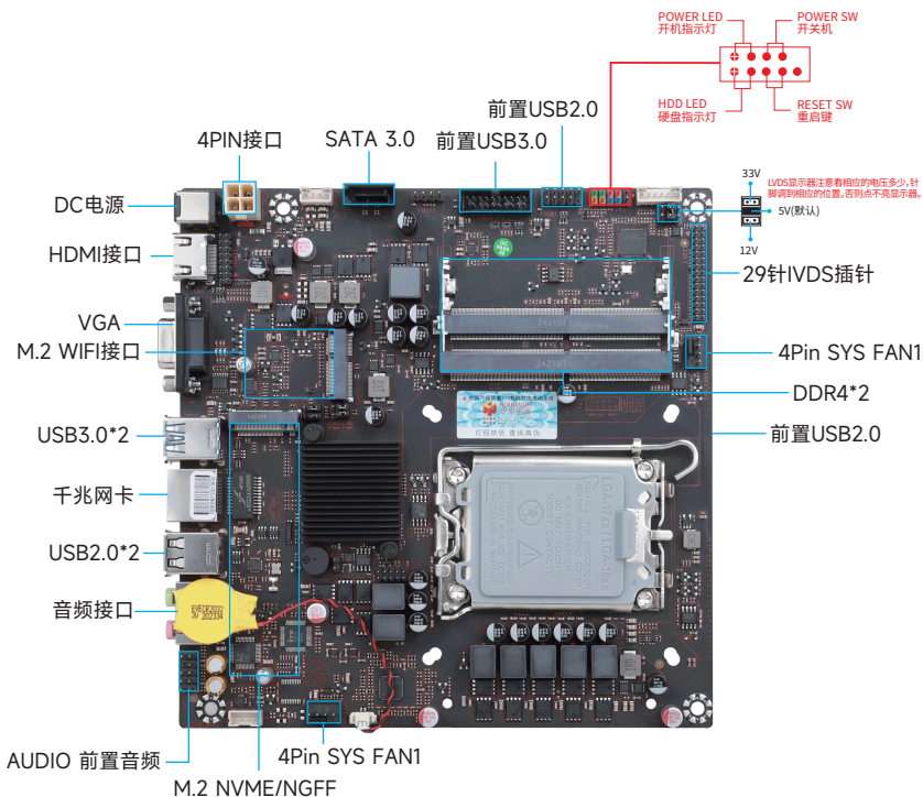
图1-1 H610M-I主板图解
