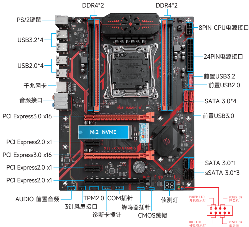
图1-1 X99-CD3 GAMING主板图解
