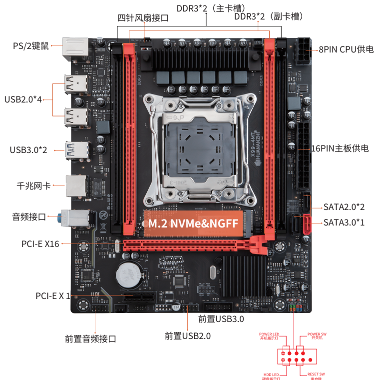
图1-1 X79-4MT V2.0主板图解
